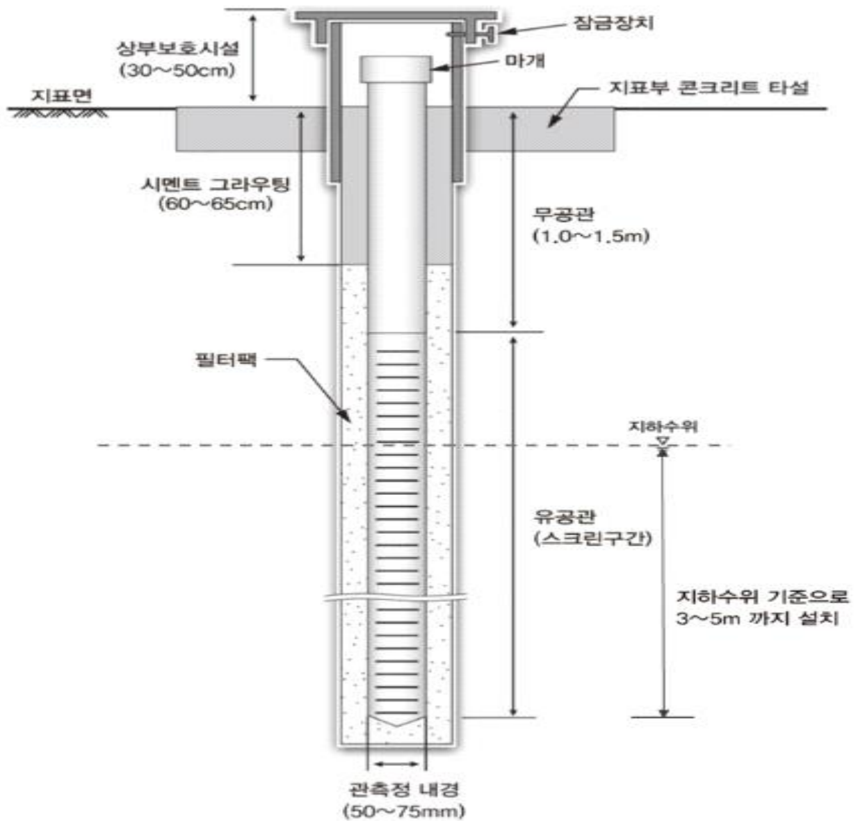
[별표 5] 관측정 구조 기본도
